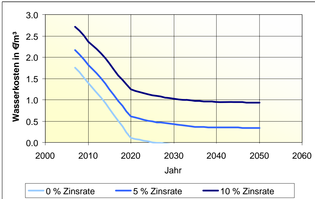
Abbildung 5: Wasserkosten für solarthermische Kraftwerke mit Multi-Effekt-Entsalzung (CSP/MED) für verschiedene Verzinsungen des Einsatzkapitals und für einen festen Stromerlös von 0.05 €/kWh. Langfristig können im Referenzfall mit 5 % Realverzinsung Wasserkosten von 0.34 €/m³ erreicht werden. Höhere Stromerlöse würden den Wasserpreis senken und umgekehrt. Angenommener Wechselkurs US$/€= 1.
