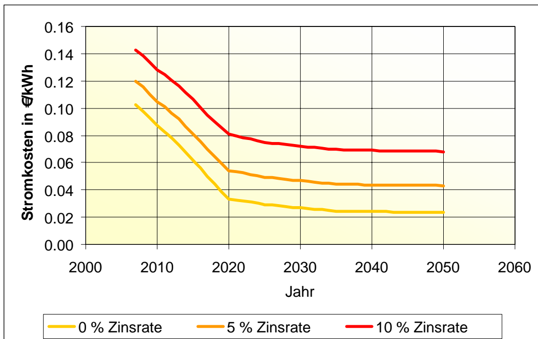
Abbildung 6: Stromkosten für solarthermische Kraftwerke mit Multi-Effekt-Entsalzung (CSP/MED) für verschiedene Verzinsungen des Einsatzkapitals und für einen festen Wassererlös von 0.5 €/m³. Langfristig können im Referenzfall mit 5 % Realverzinsung Stromkosten von 0.04 €/kWh erreicht werden. Höhere Wassererlöse würden den Strompreis senken und umgekehrt. Angenommener Wechselkurs US$/€= 1.
